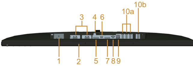
Monitör standı olmadan arkadan görünüm
